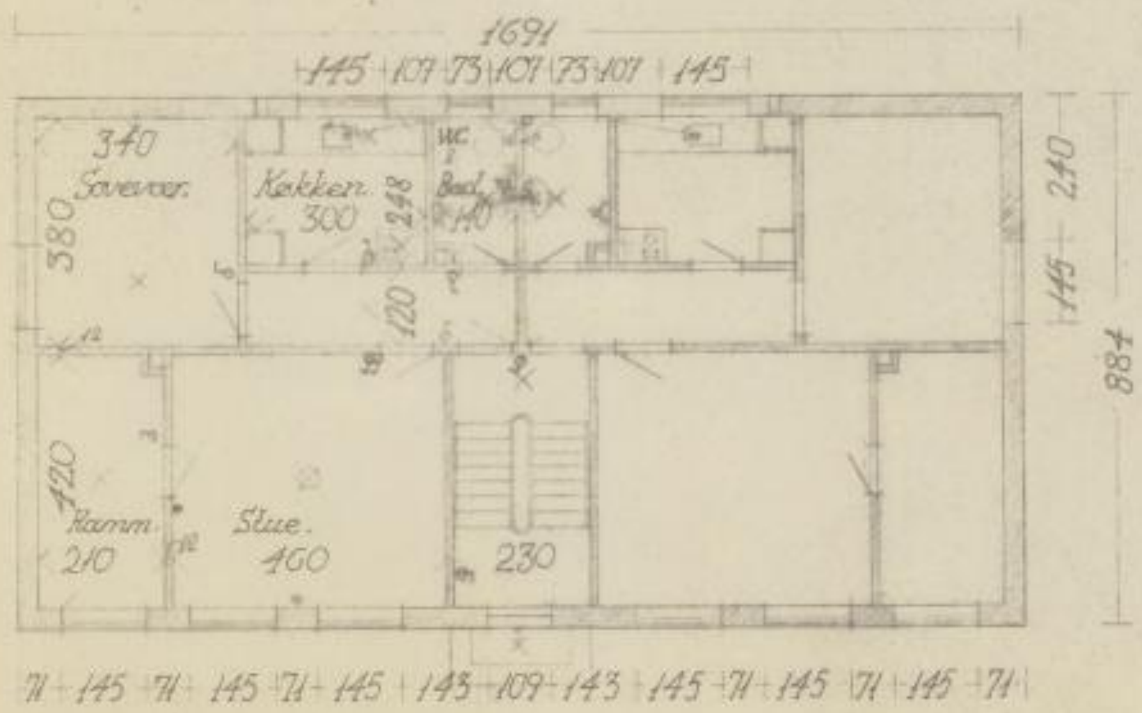
Etageplan.
