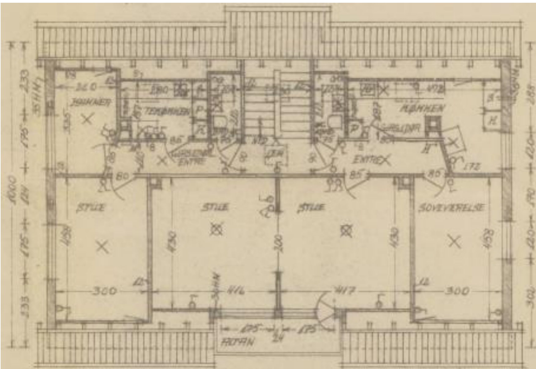
LOFTPLAN
